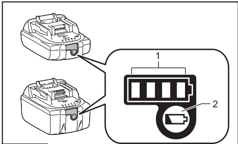
Fig.2 ► 1. Témoins indicateurs 2. Bouton de vérification
