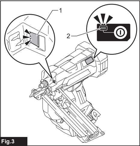
Fig.3 ► 1. Lampe 2. Voyant d'alimentation
