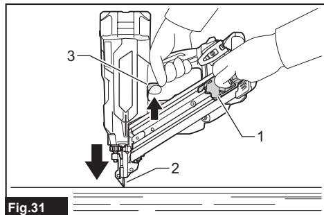
► 1. Palanca pulsadora 2. Elemento de contacto 3. Gatillo interruptor
