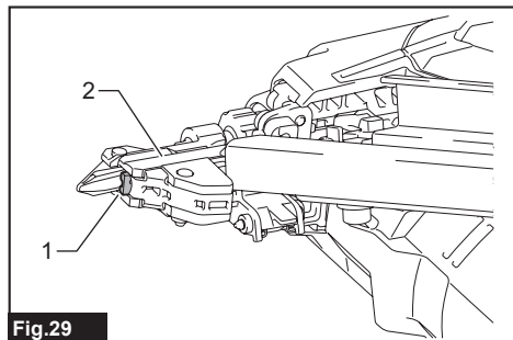
► 1. Impulsor 2. Guía del impulsor
